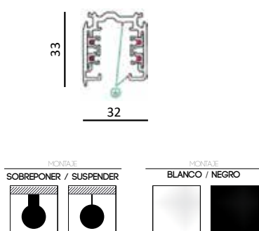
RIEL DE ALUMINIO 3 CIRCUITOS 3 M MODELO: 51072
