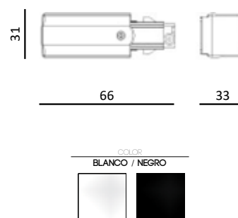
CONECTOR DE ALIMENTACIÓN PARA RIEL DE 3 CIRCUITOS MODELO: 51182
