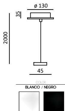
ACCESORIO PARA SUSPENDER RIEL DE 3 CIRCUITOS MODELO: 51302
