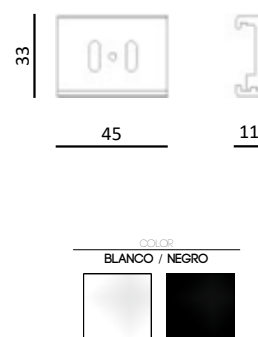
ACCESORIO PARA SOBREPONER RIEL DE 3 CIRCUITOS MODELO: 51222
